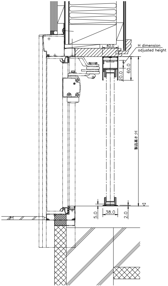
Zipooh (88LME) Longitudinal section
