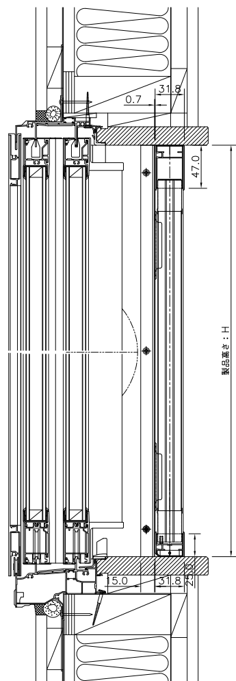
インテリア網戸 正面付 縦断面図
