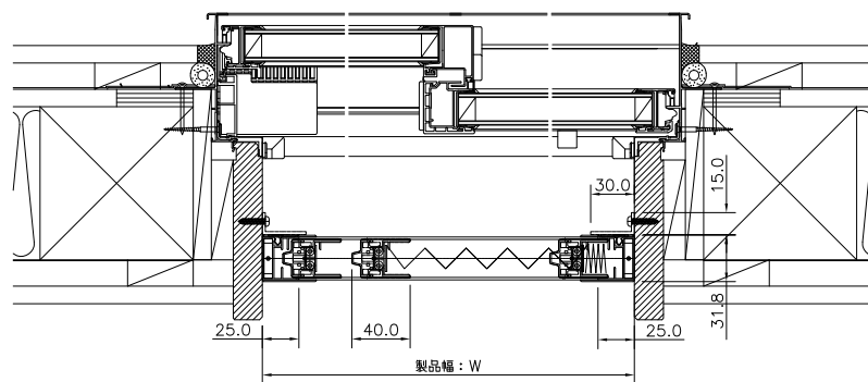
インテリア網戸 正面付 片引き 横断面図
