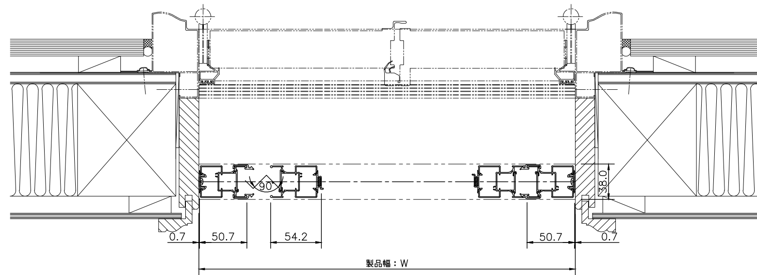
侍風 両引き (88LME) 横断面図
