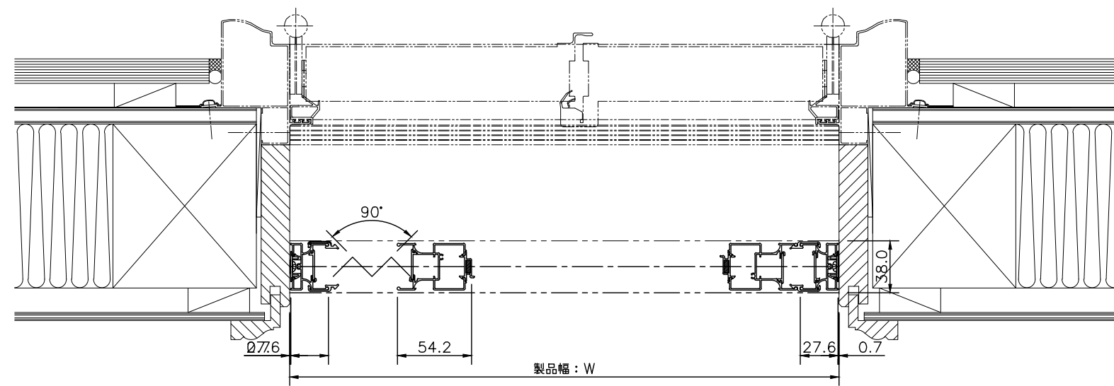
侍風 両引き (8LME) 横断面図
