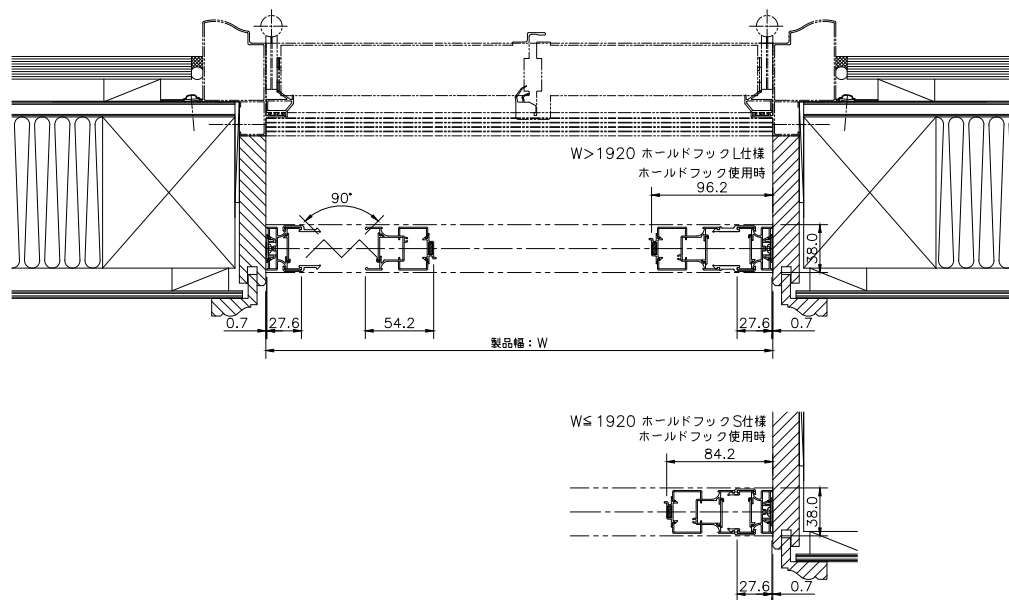
侍風 両引き (8LME) 横断面図
