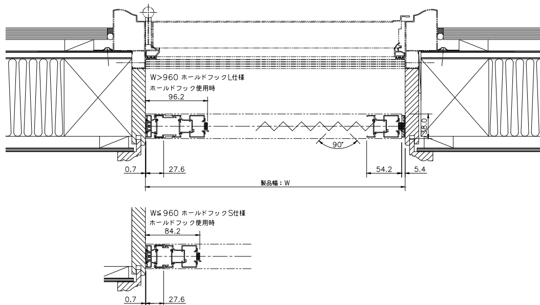
侍風 片引き (8LME) 横断面図
