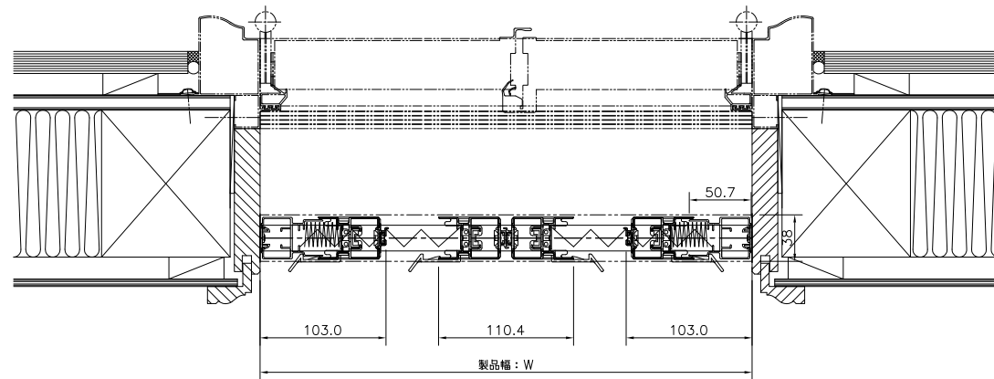
ぎやたぴら網戸2 両引き (88L) 横断面図
