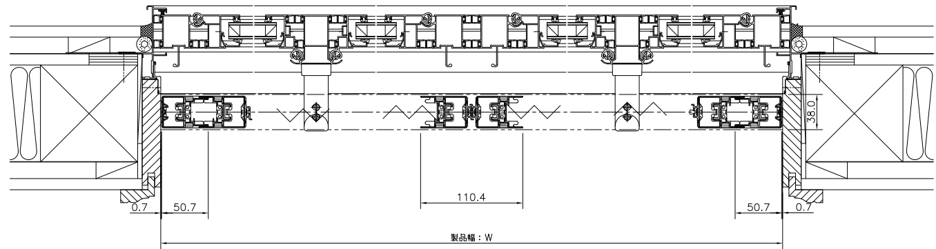
ぎやたぴら網戸2 両引き (88LW) 横断面図
