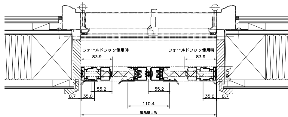
ぎゃたびら網戸2 両引き (8LF) 横断面図
