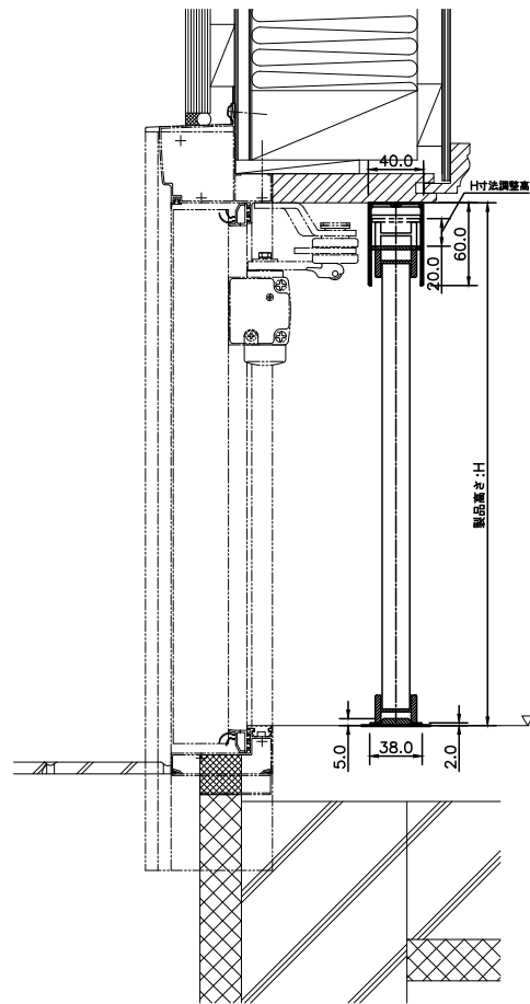
ぎゃたびら網戸2 (8LF) 縦断面図
