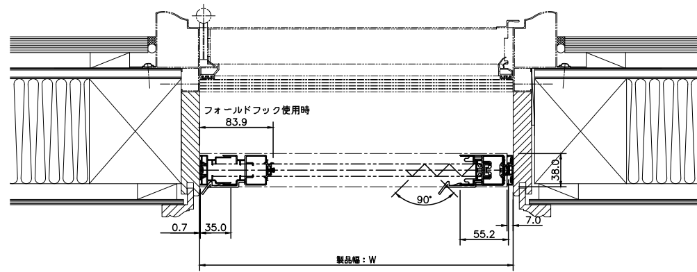
ぎゃたびら網戸2 片引き (8LF) 横断面図
