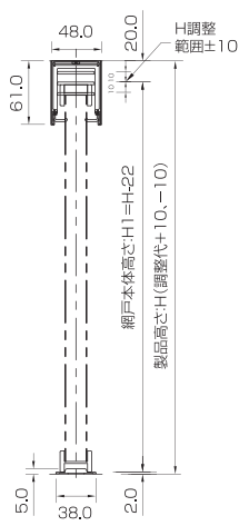
● 両引き (3+3)枚建て
