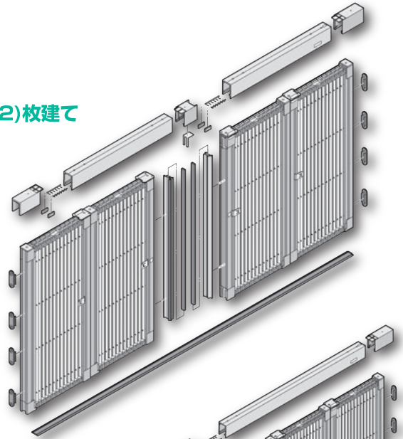
● 両引き (3+3)枚建て
