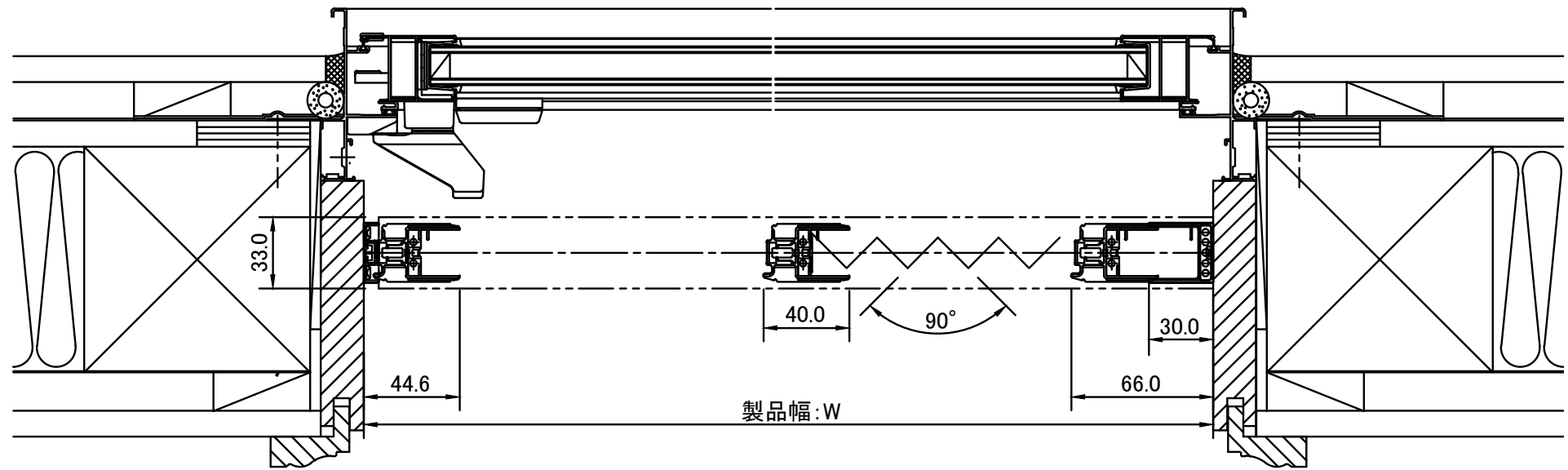
プリーツシェード 片引き(20mm)横断面図
